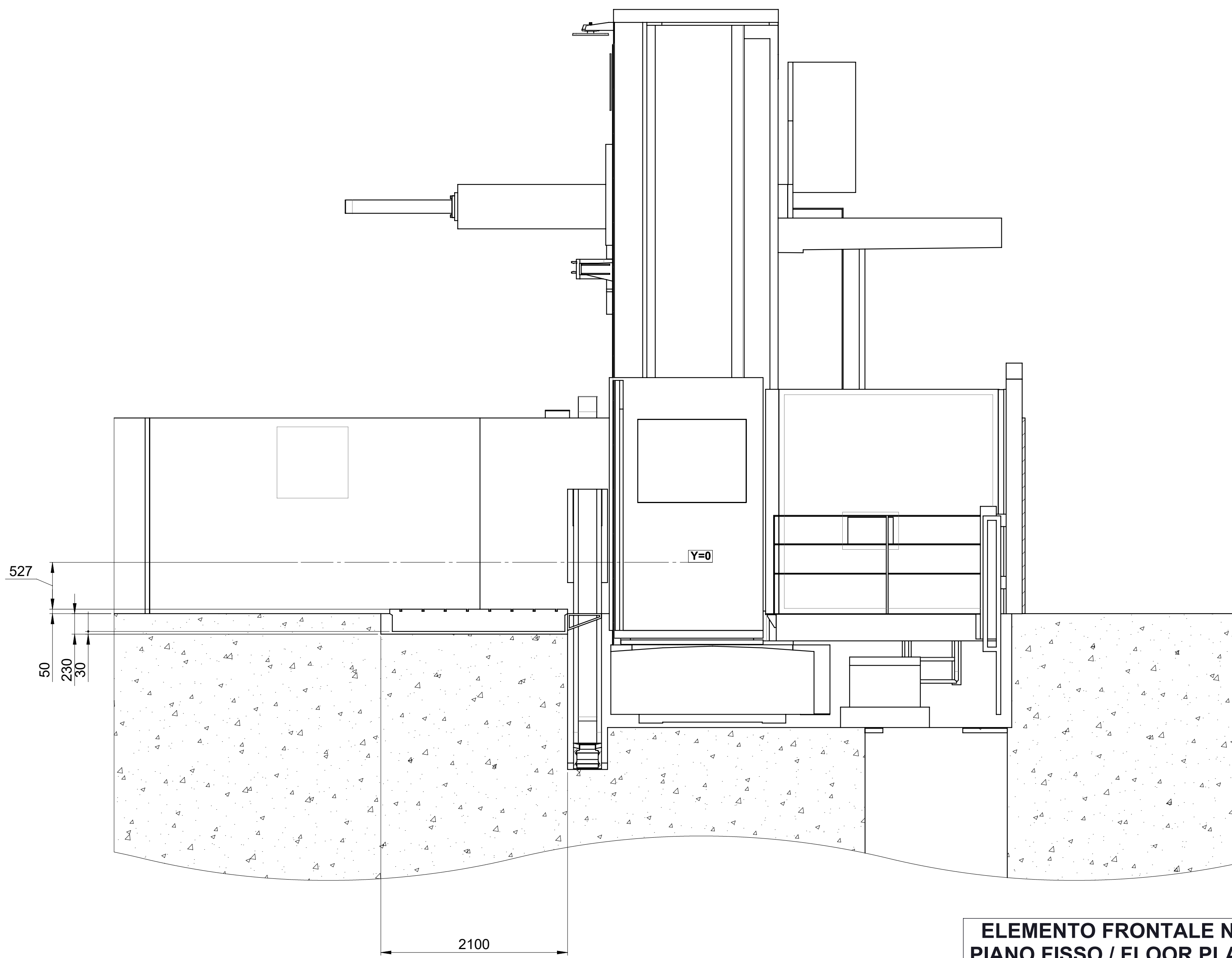
C-C 270°
