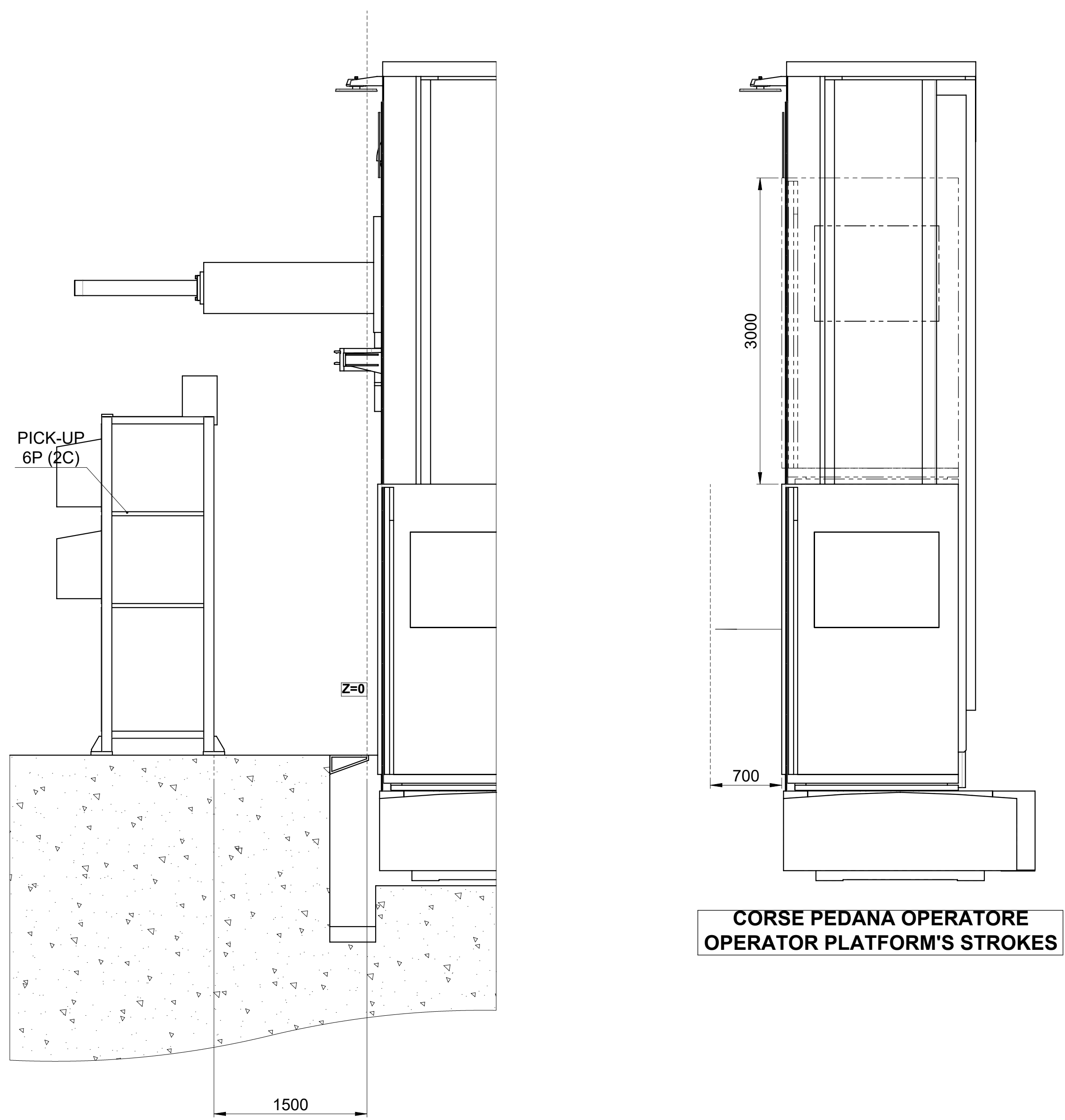
A-A 270°
